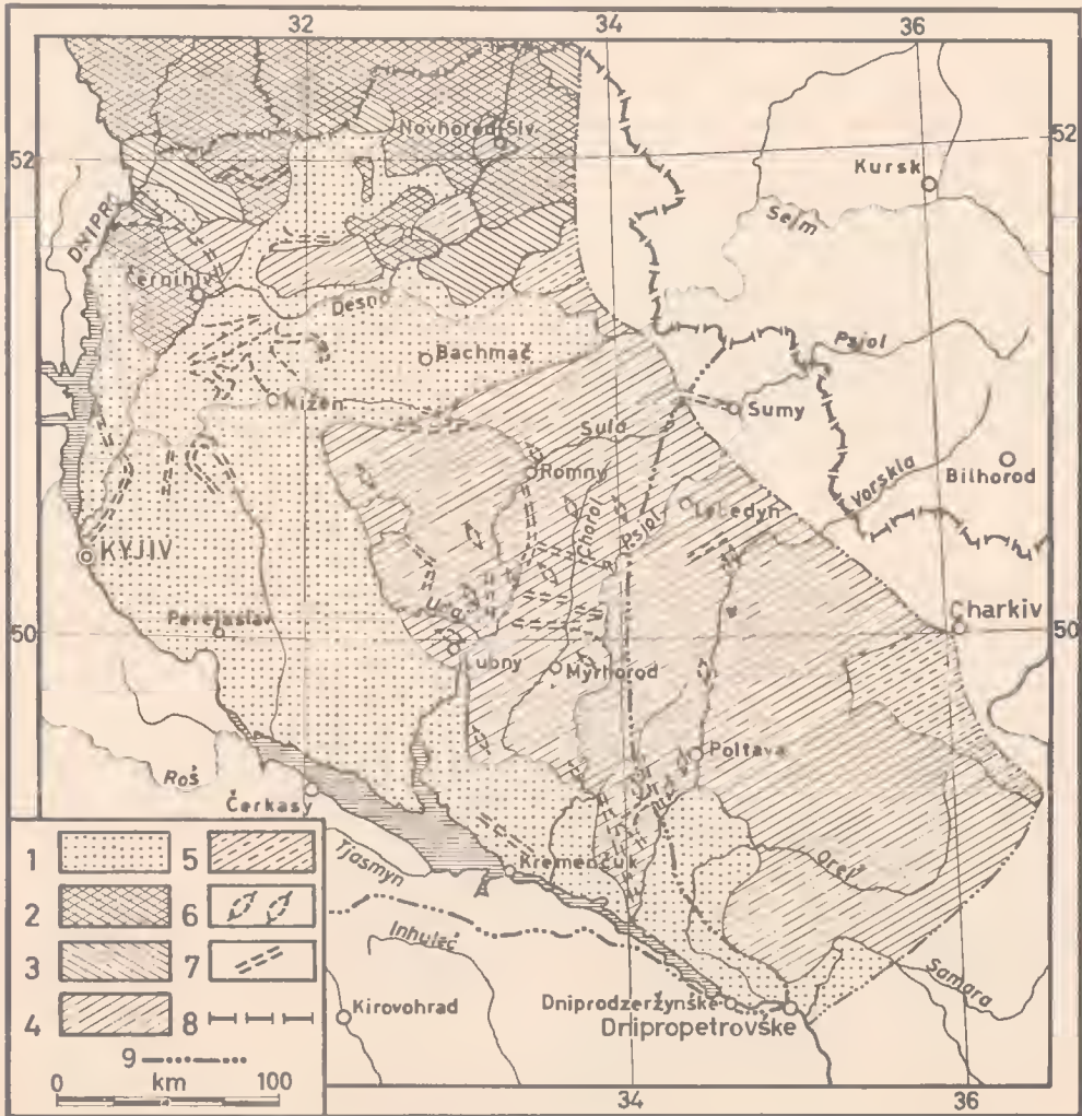
Геоморфологічна карта Придніпровської низовини
